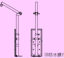
SB防水腰壁付型
